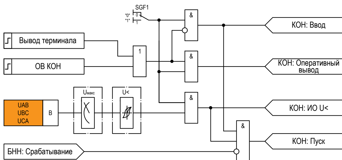
Рисунок 2.23 – Функциональная схема «КОН»
