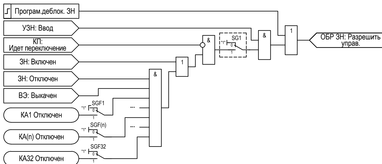
Рисунок 2.33 – Функциональная схема «ОБР ЗН»
